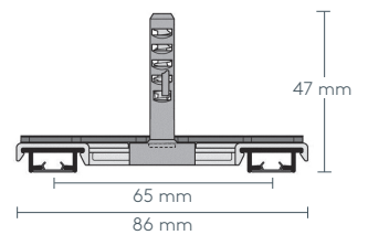
2-Lauf-Adapter mit Klick-Deckenträger für zweiläufige Garnitur
