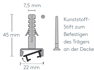
Klick-Deckenträger mit Stift für einläufige Garnitur
