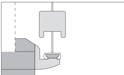
Schnitt Fensterrahmen mit Kunststoffträger und Unterschiene
