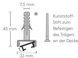
Klick-Deckenträger mit Stift für einläufige Garnitur
